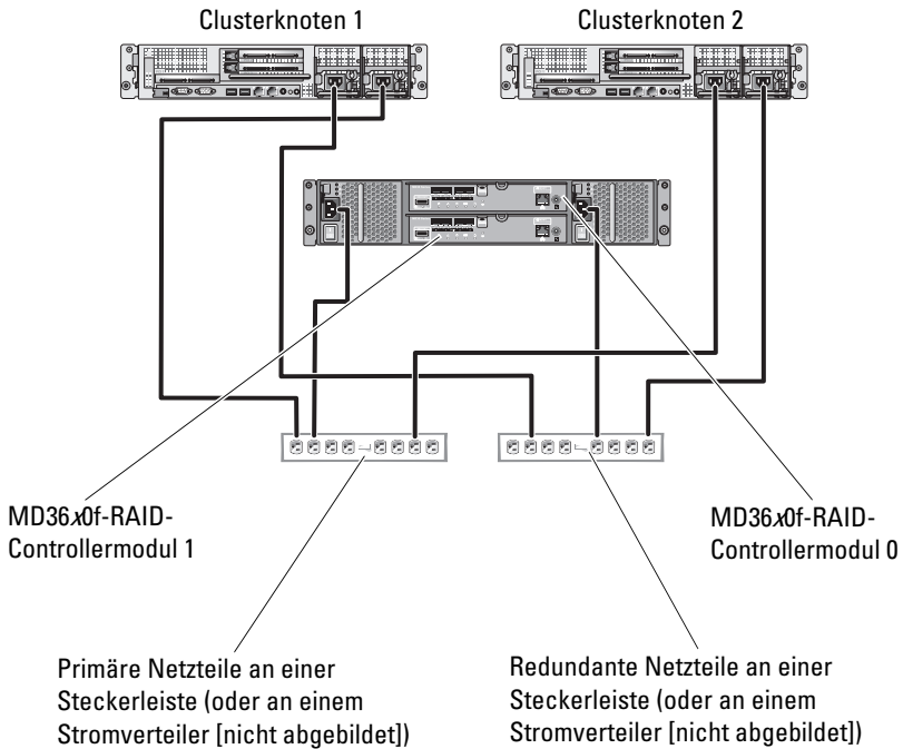
Abbildung 2-1. Beispiel für die elektrische Verkabelung
