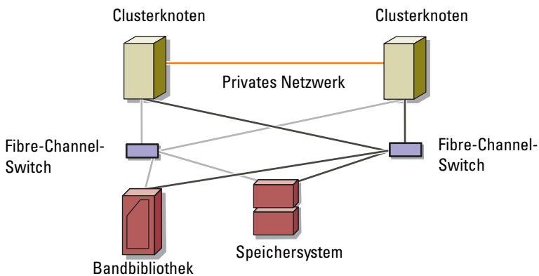
Abbildung 2-9. Speichersystem mit einer Bandbibliothek verkabeln
