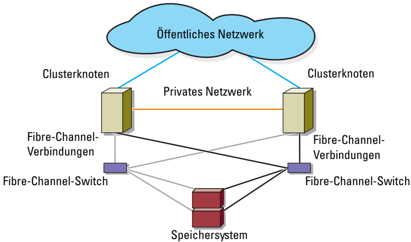
Abbildung 1-2. SAN-Attach-Cluster
