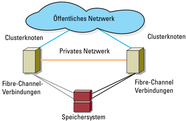
Abbildung 1-1. Direct-Attach-Konfiguration mit einem einzelnen Cluster
