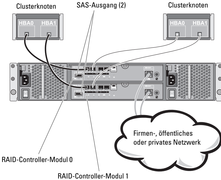
Abbildung 2-4. Verkabelung eines Direct-Attached-Clusters mit zwei Knoten mit einem PowerVault MD36x0f-Speichersystem
