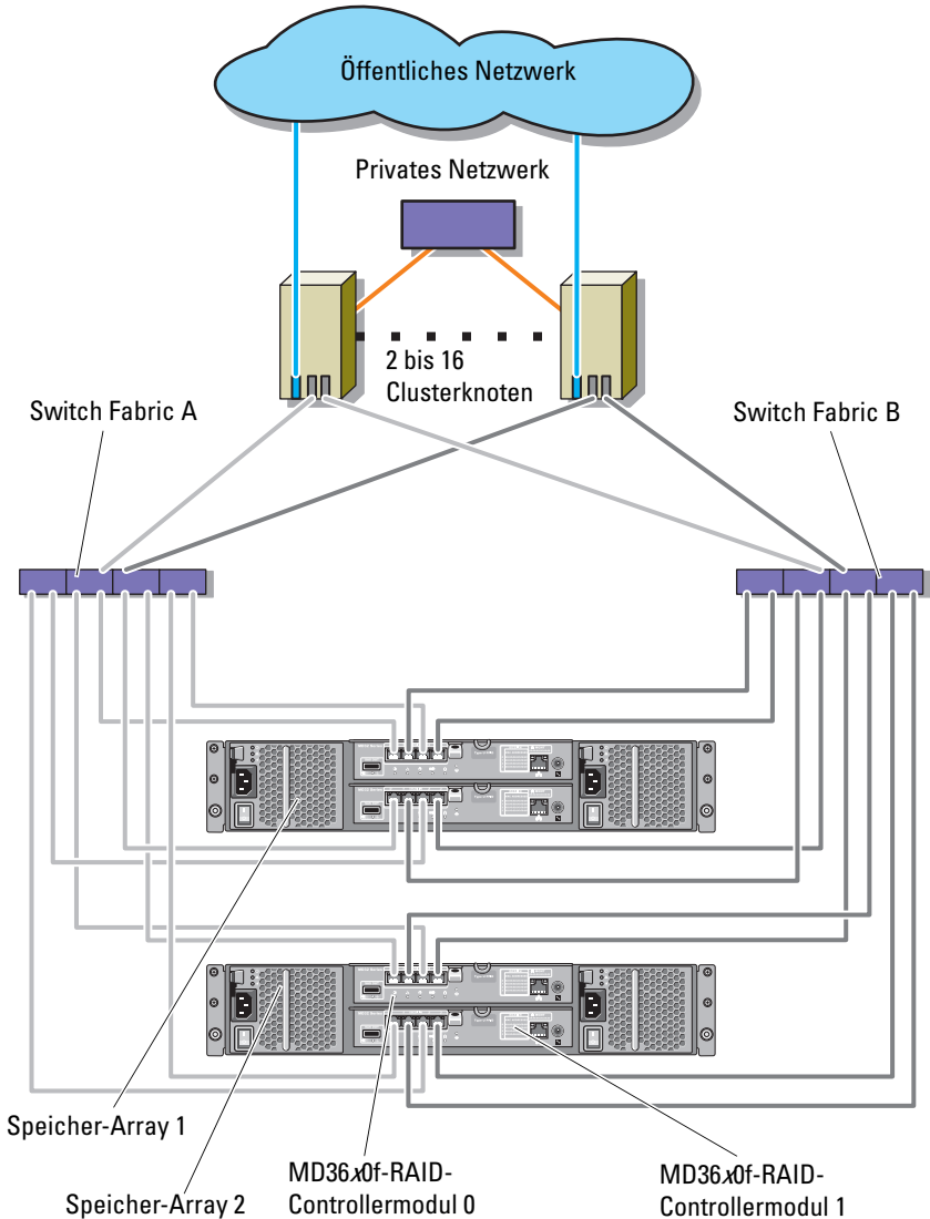
Abbildung 2-10. Network-Attached-Clusterkonfiguration mit mehreren Speicher-Arrays
