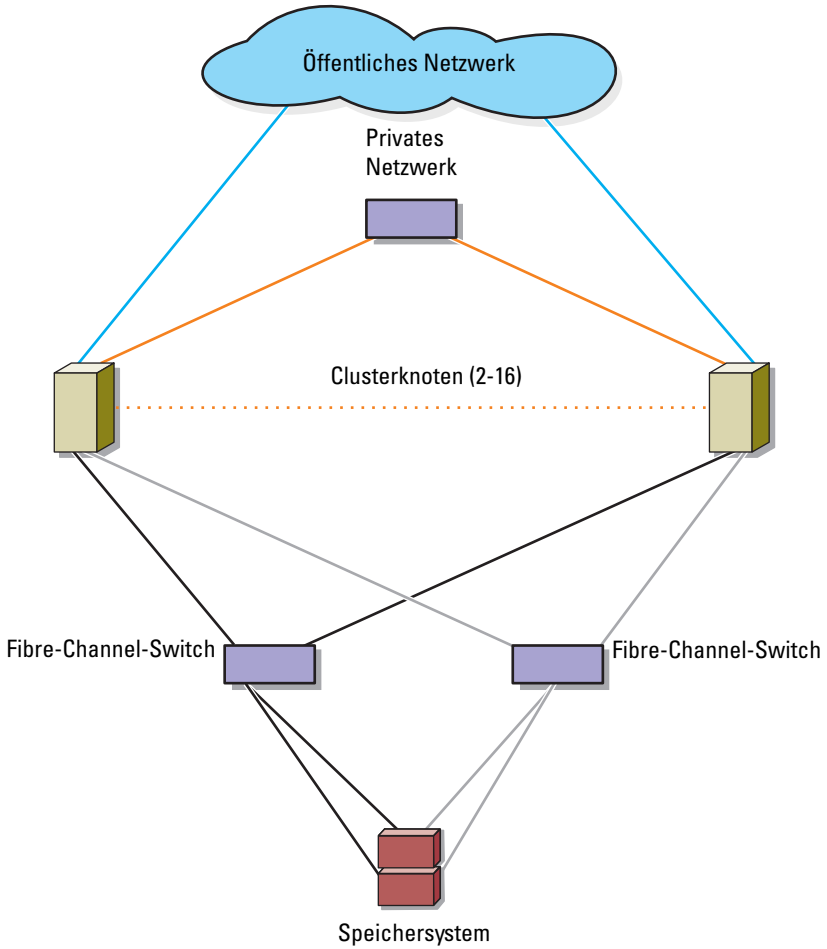
Abbildung 2-7. SAN-Attach-Cluster mit sechzehn Knoten
