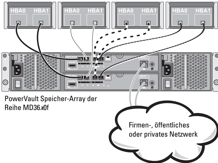
Abbildung 2-5. Verkabelung eines Direct-Attached-Clusters mit vier Knoten mit einem PowerVault MD36x0f-Speichersystem
