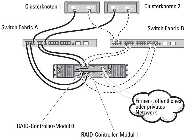
Abbildung 2-8. Verkabelung eines SAN-Attached-Clusters mit dem MD36x0f
